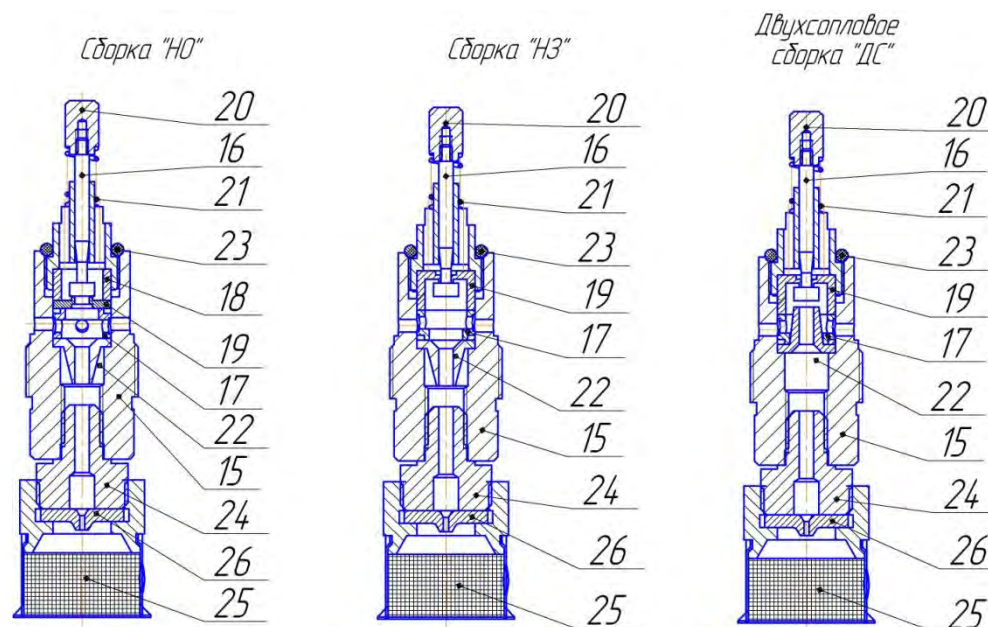
Рис 3. - Управляющие клапанки
